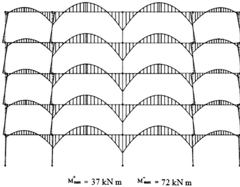
Fig. E15.1e Moment diagram for uniform loading
