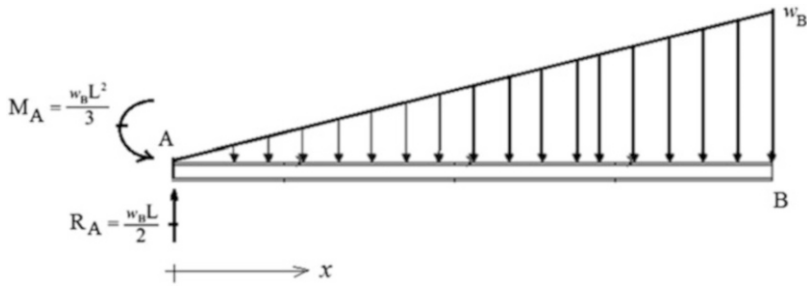
Fig. E3.10b Reactions
