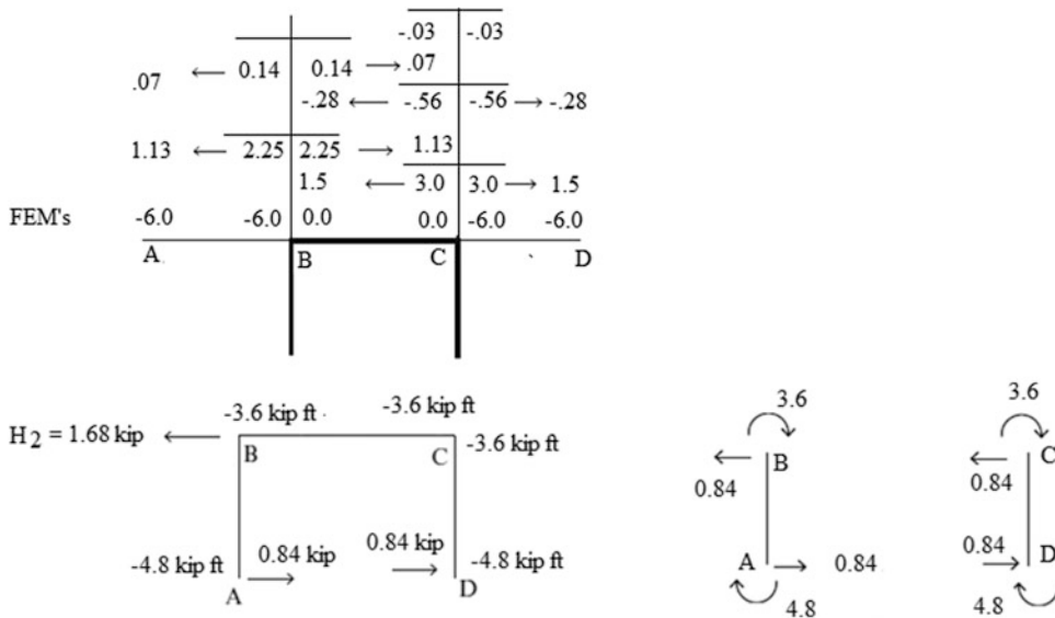
Fig. E10.17e Case II—end moments and column shear
