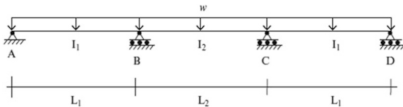
Fig. E10.5a Uniform load
