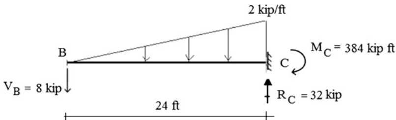
Fig. E3.13c Segment BC
