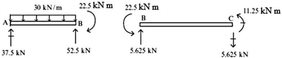
Fig. E10.10b Free body diagrams
