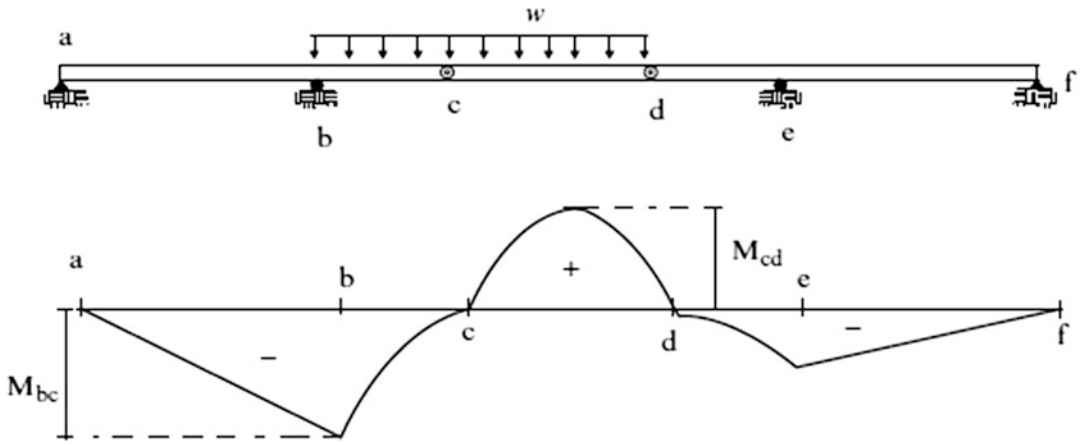
Fig. E3.28d Moment diagram
