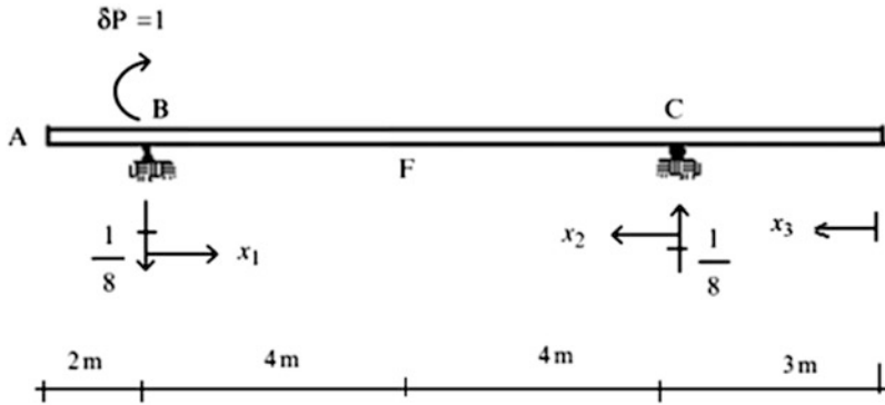
Fig. E3.24d \delta M_{\theta_B}(x)
