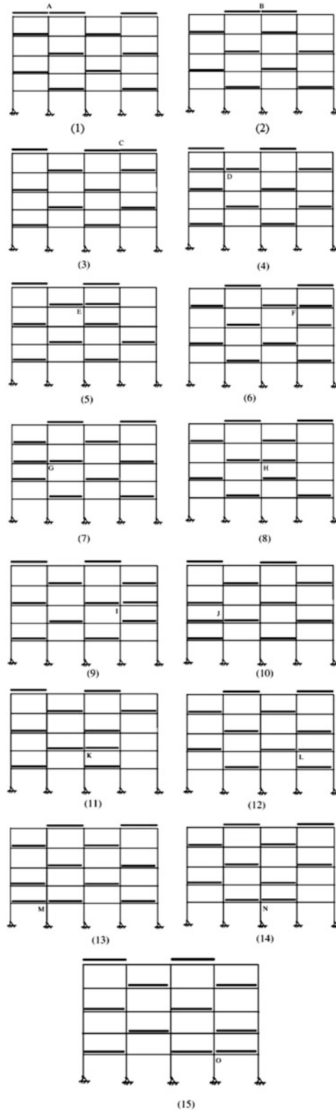
Fig. E15.1c Live load patterns for negative moment
