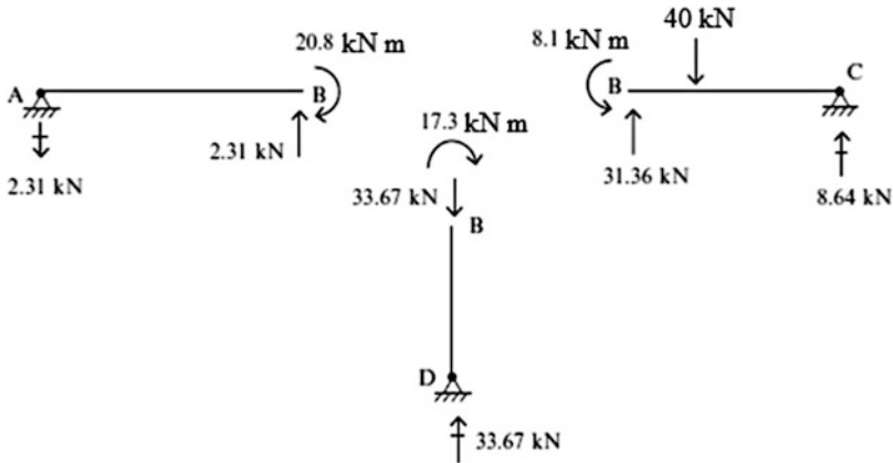
Fig. E10.7c Free body diagrams
