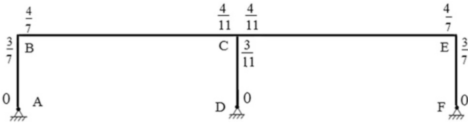
Fig. E10.14b Distribution factors
