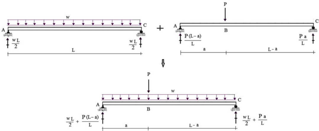
Fig. E3.11b Reactions
