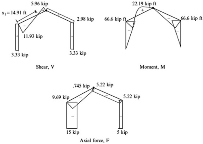
Fig. E4.10e Shear and moment diagrams
