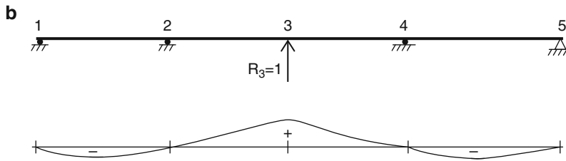
Fig. E13.1b Influence line for R_3
