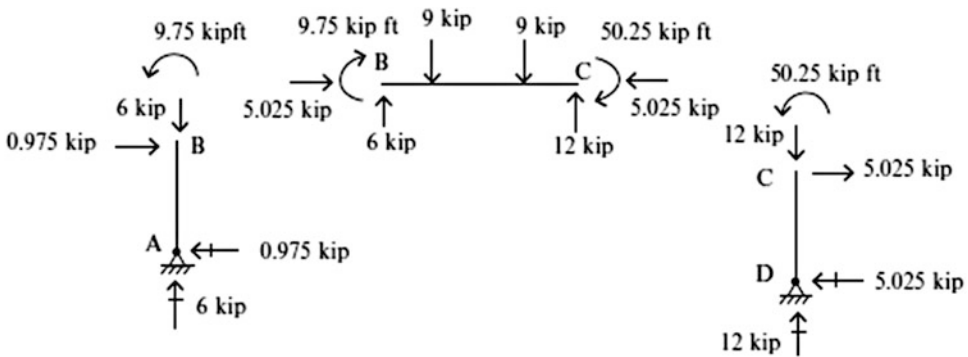
Fig. E10.8d Free body diagrams
