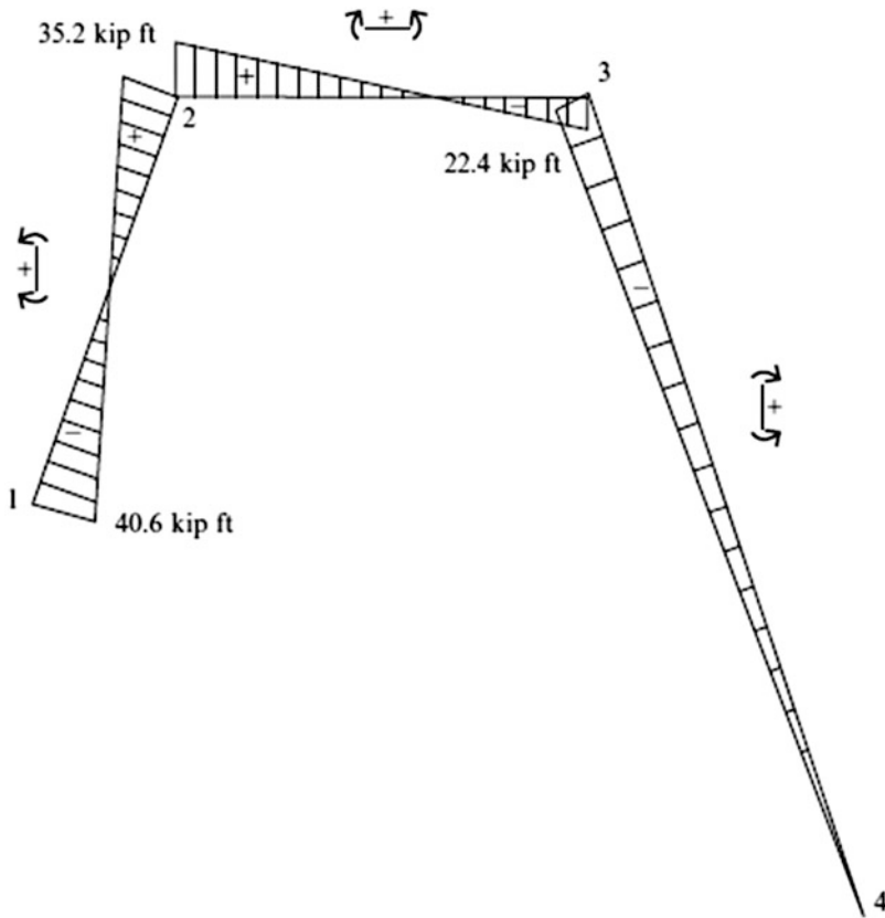
Fig. E10.19e Moment diagram
