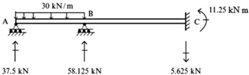
Fig. E10.10c Reactions
