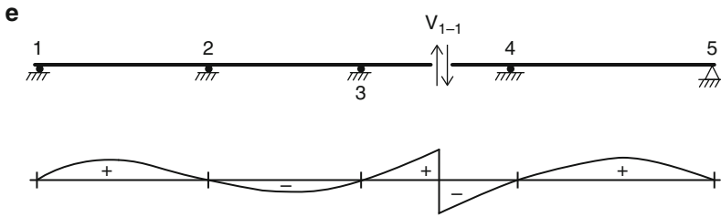
Fig. E13.1e Influence line for V_{1-1}
