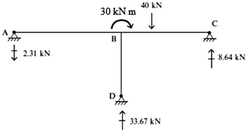
Fig. E10.7d Reactions
