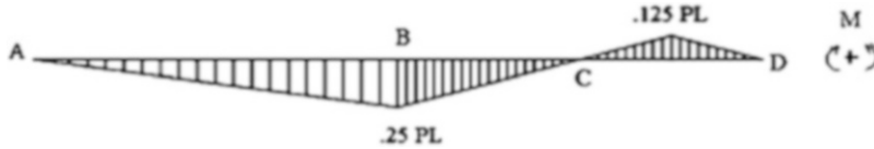
Fig. E3.18b Moment diagram
