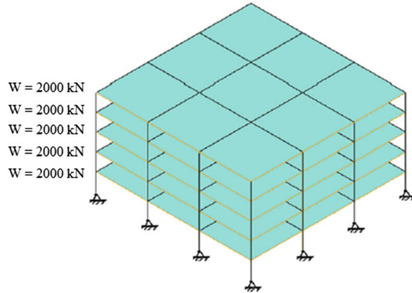
Fig. E15.2a 3D model
