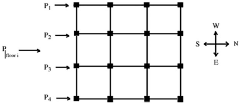
Fig. E14.16d Floor load distribution
