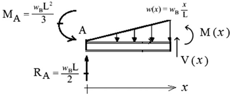
Fig. E3.10b Reactions
