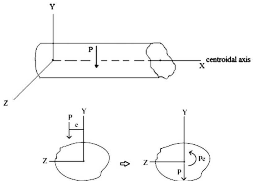
Fig. 3.34 Prismatic member—eccentric load
