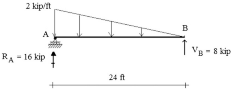
Fig. E3.13b Segment AB
