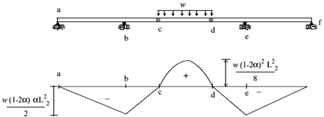
Fig. E3.28e Moment diagram
