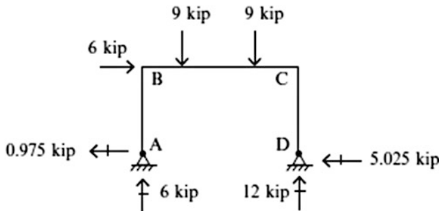
Fig. E10.8d Free body diagrams
