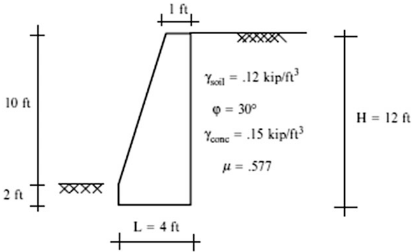
Fig. E8.1a Wall geometry
