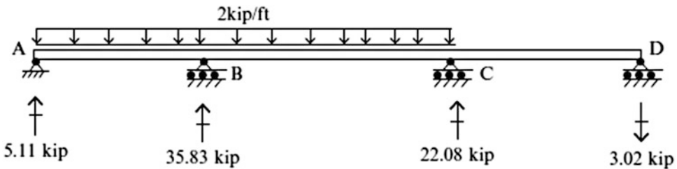
Fig. E10.12c Reactions
